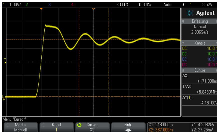
Abbildung 29 Cursor messen Überschwingfrequenz
